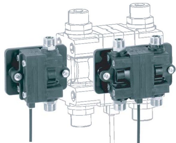
IF01 Einzelventil
